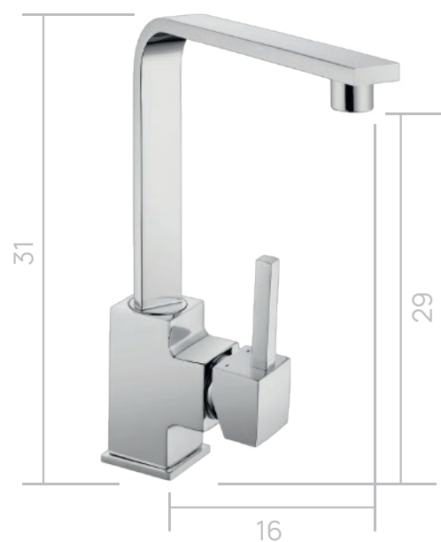
BICA MÓVEL CÓDIGO: 2139
