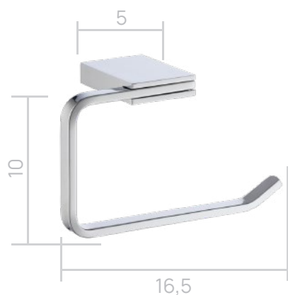
PORTA PAPEL HIGIÊNICO CÓDIGO: 40251
