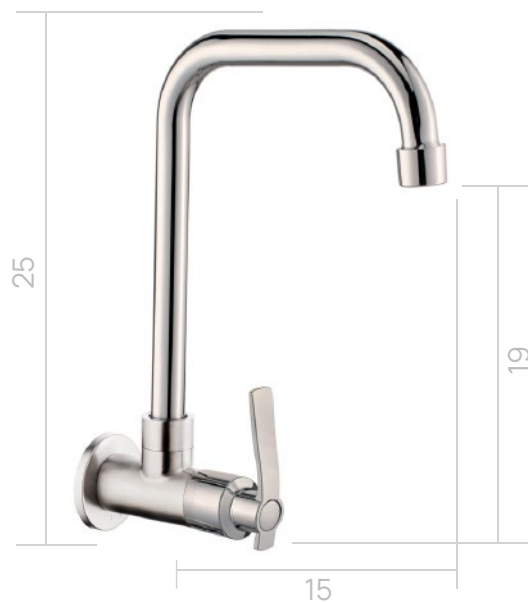
INOX POLIDO CÓDIGO: 9935
