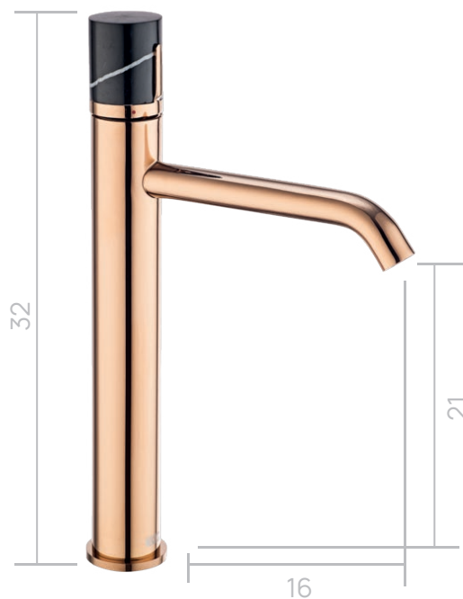
MANOPLA MÁRMORE PRETO CÓDIGO: 1662
